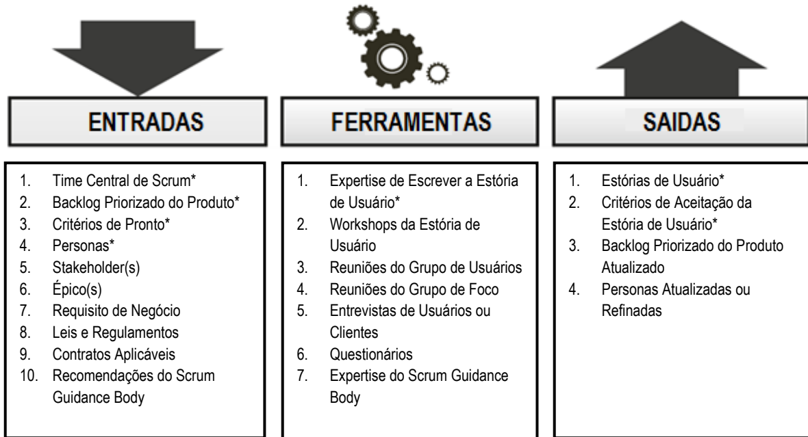
Figura 9-3: Criar as Estórias de Usuário—Entradas, Ferramentas, e Saídas
