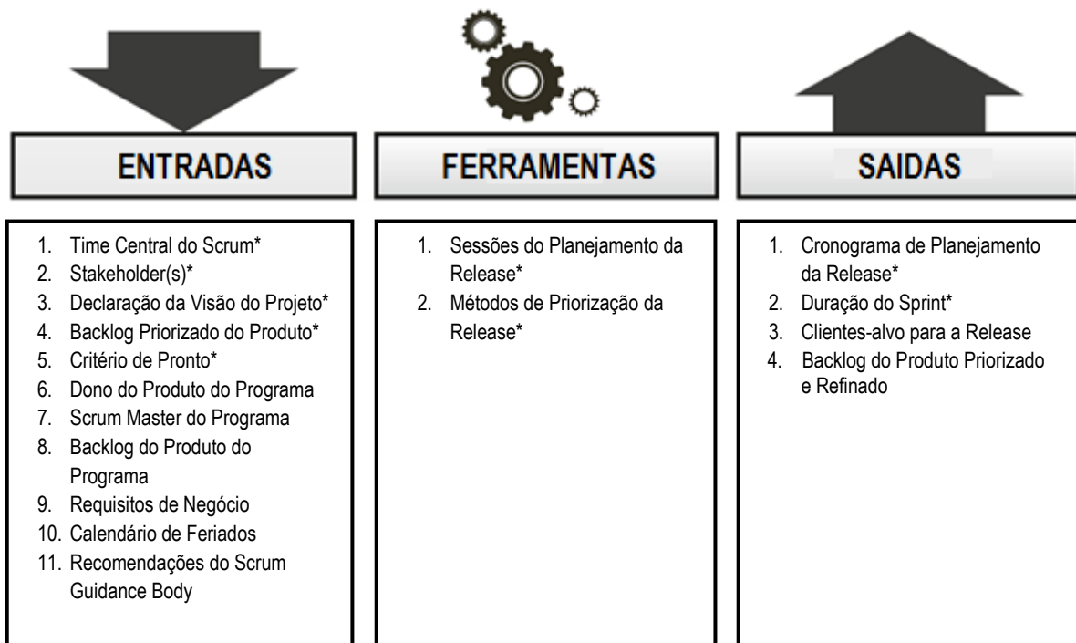
Figura 8-9: Conduzir o Planejamento de Release—Entradas, Ferramentas, e Saídas
