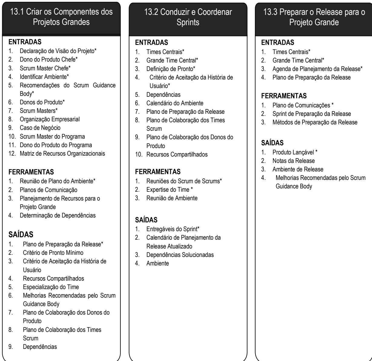
Figure 13-1: Overview do Scrum em Escala para Projetos Grandes
