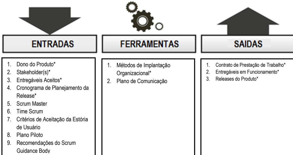
Figura 12-3: Envio de Entregáveis—Entradas, Ferramentas, e Saídas
