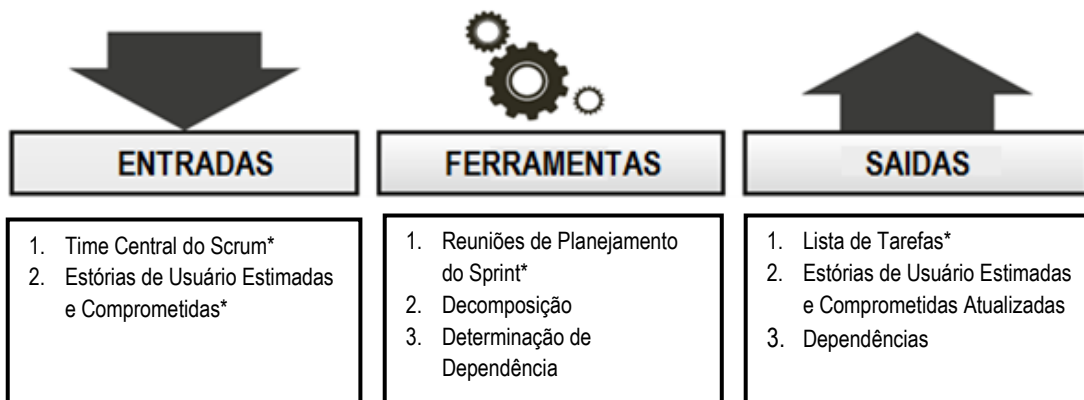
Figura 9-6: Identificar as Tarefas—Entradas, Ferramentas, e Saídas
