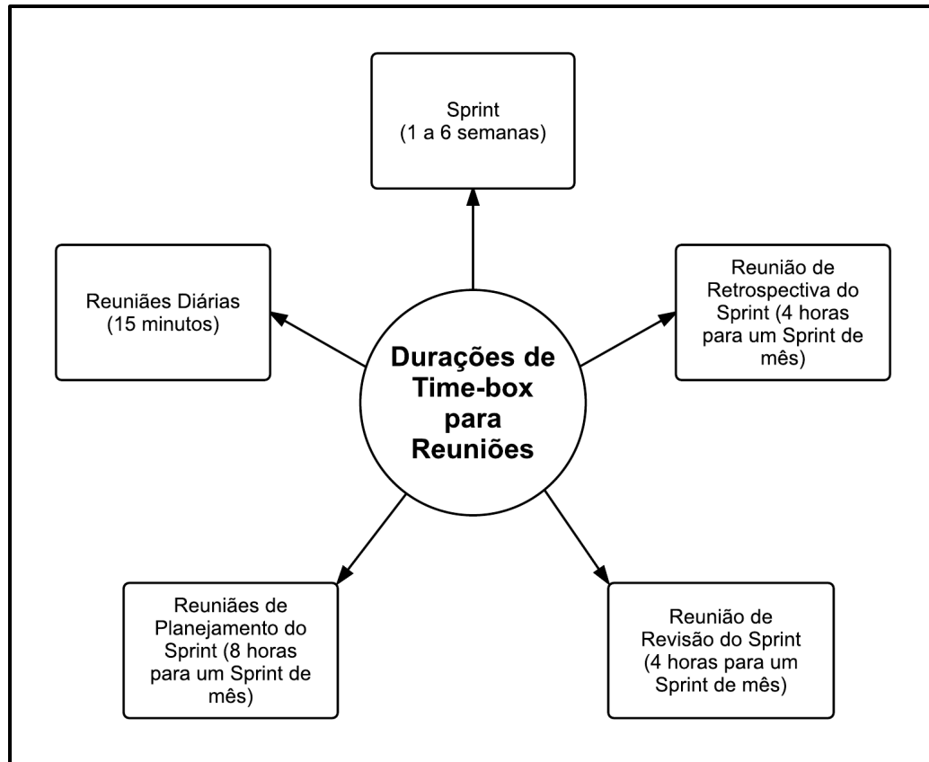
Figura 2-8: Durações Time-Box para Reuniões do Scrum
