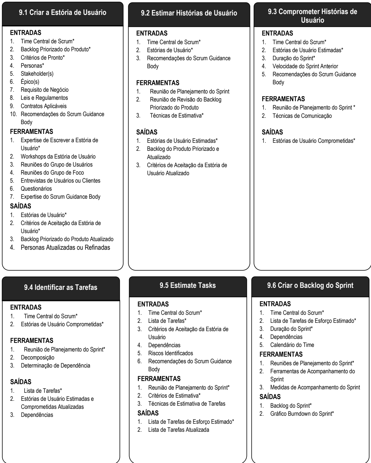
Figura 9-1: Visão Geral de Planejar e Estimar
