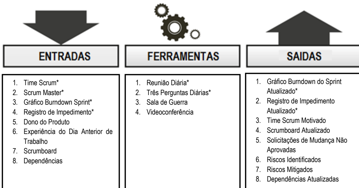
Figura 10-5: Conduzir a Reunião Diária—Entradas, Ferramentas, e Saídas
