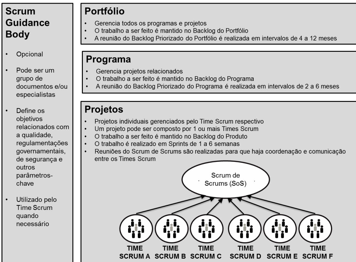
Figura 3-4: Scrum em Toda a Organização para Projetos, Programas e Portfólios
