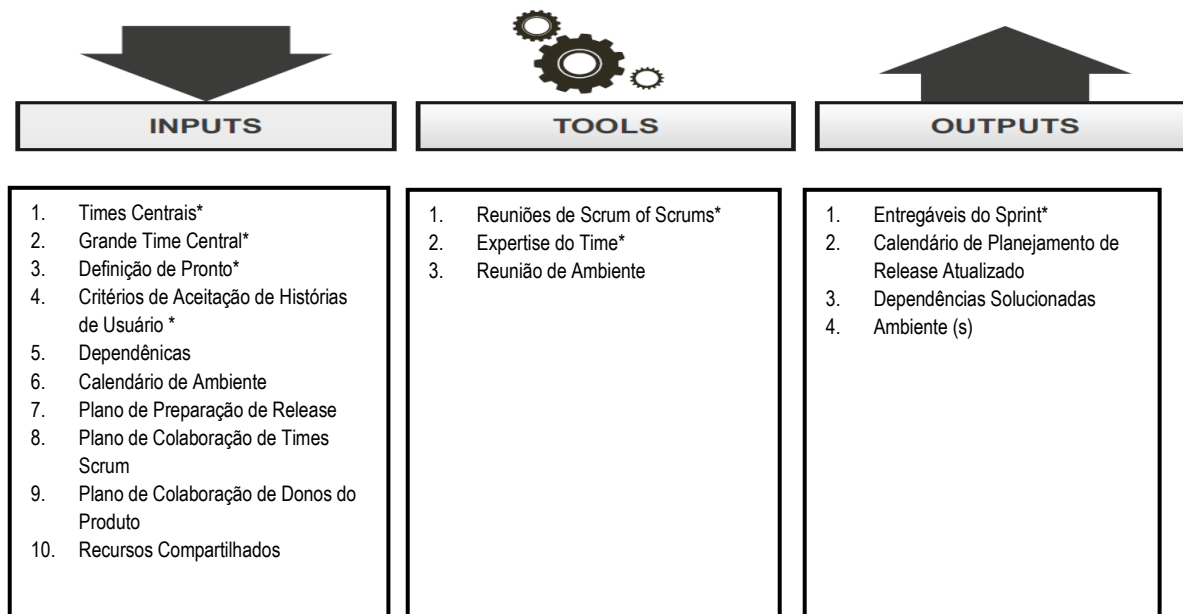
Figura 13-3: Conduzir e Coordenar Sprints – Entradas, Ferramentas e Saídas
