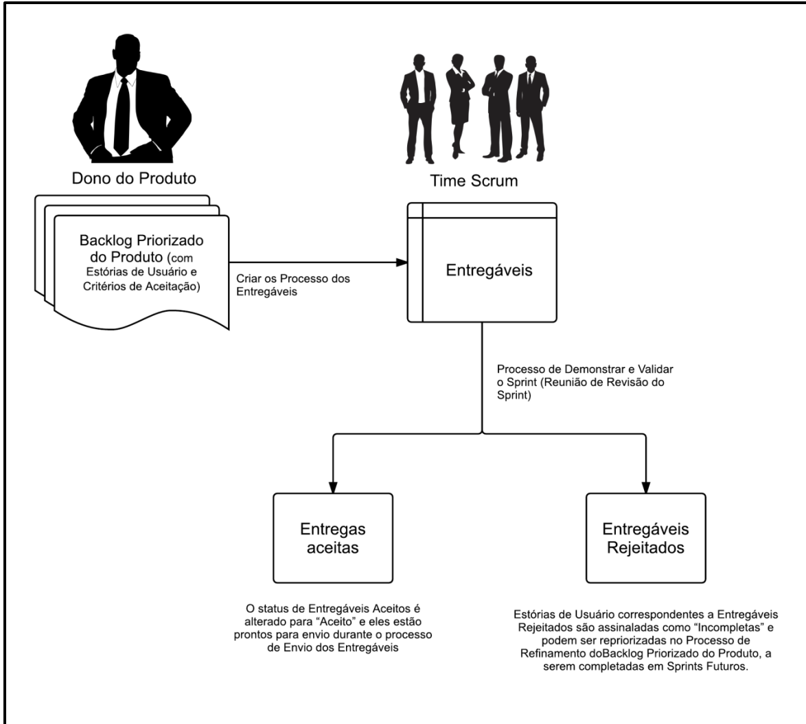
Figura 5-1: Diagrama de Fluxo de Incremento do Projeto
