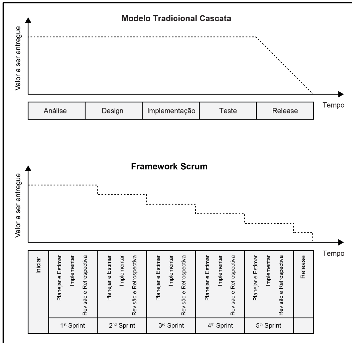
Figura 2-9: Scrum x O Modelo Tradicional Cascata (Waterfall)
