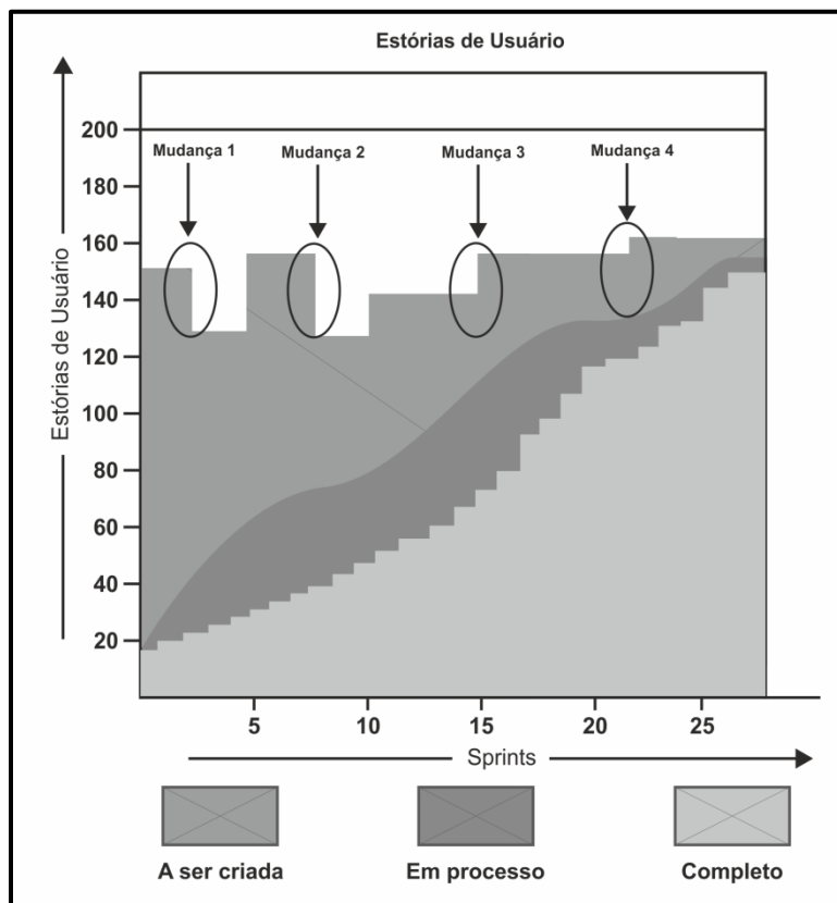
Figura 4-5: Exemplo do Diagrama de Fluxo Cumulativo (DFC)
