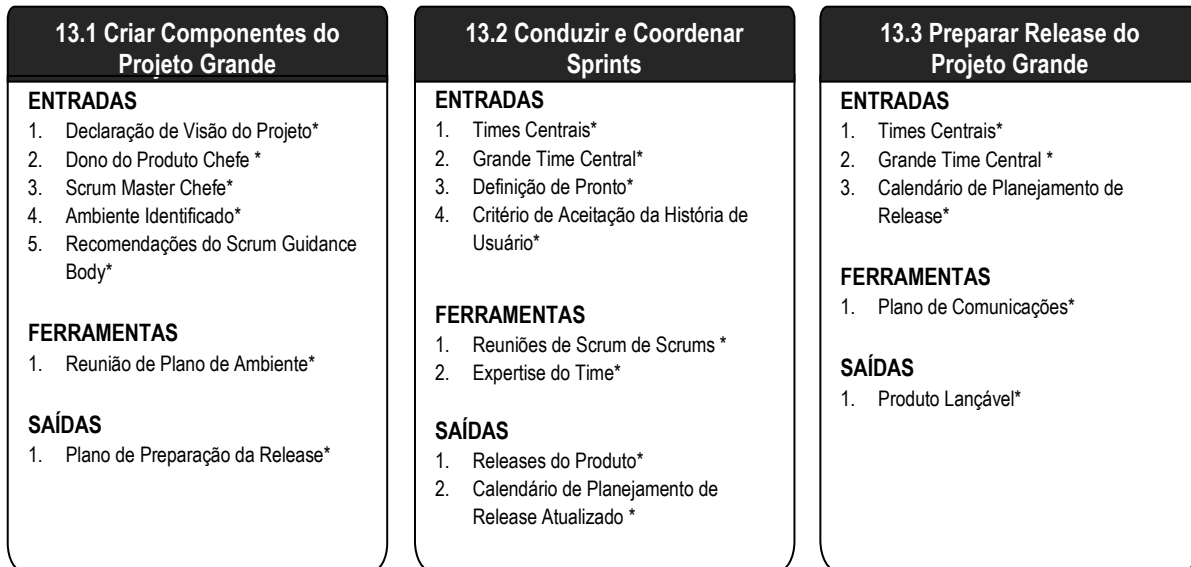
Figura 13-2: Scrum em Escala para Projetos Grandes
